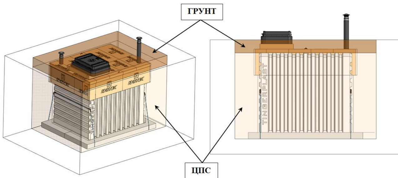
Рисунок 10 – Засыпка погреба
